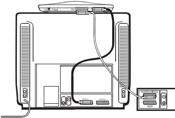
Afbeelding 18: Andere televisieapparatuur aansluiten.
